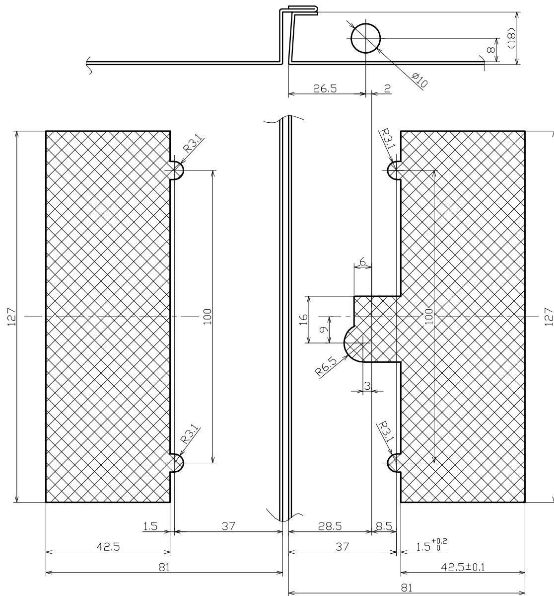
取付穴寸法
